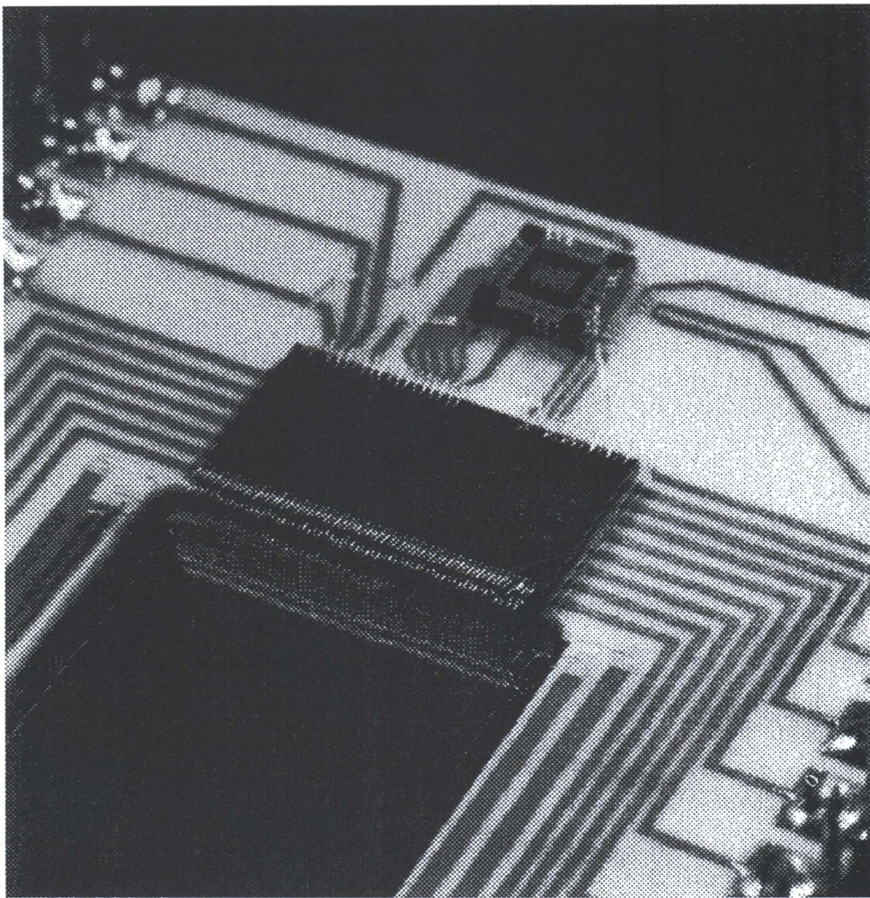
Abb.: Prototyp der Röntgen-CCD-Kamera für die Röntgensatelliten XMM und ABRIXAS.
