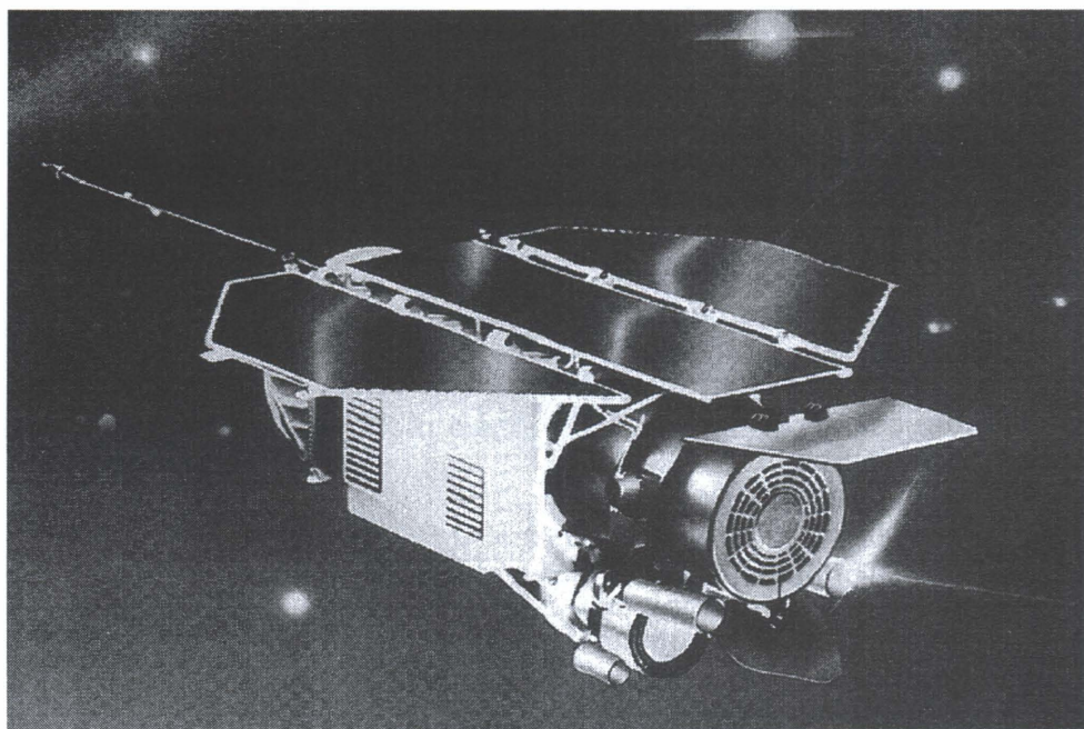
Der Röntgensatellit ROSAT des Garching MPI für Extraterrestrische Physik in der Umlaufbahn. Grafik: Dornier
